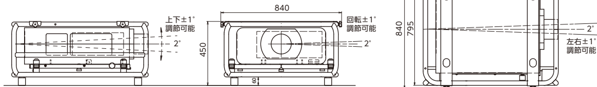
外形寸法図 (単位:mm)
